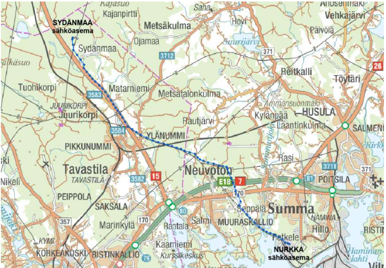
Sydänmaa-Nurkka 2x110 kV johdon sijaintikartta. Uusi voimajohto ja suunnitellut pylväspaikat merkitty sinisellä värillä
