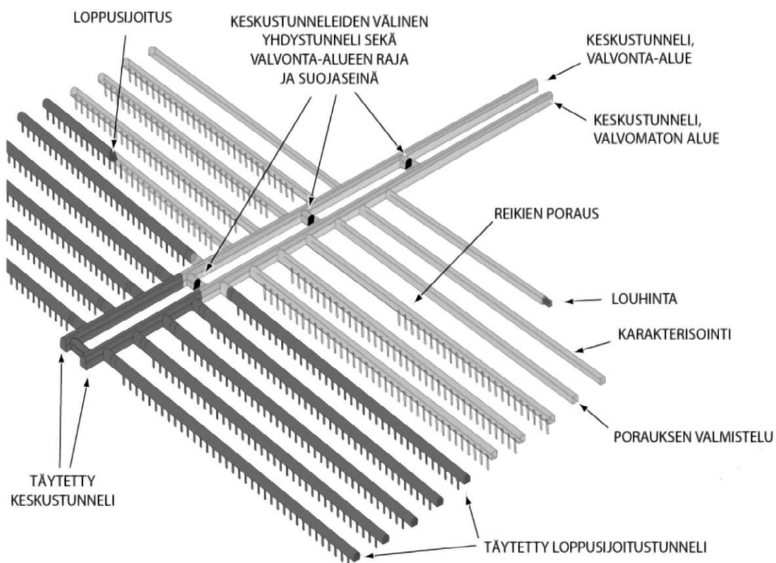
Kuva 8. Rinnakkaistunneliperiaatteella mahdollistetaan mm. parempi käytettävyys ja palo-osastointi.
