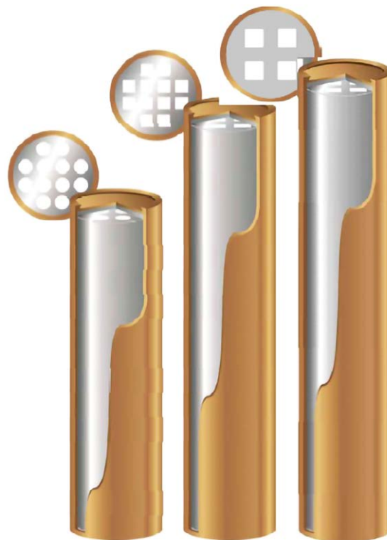
■ Kuva 4. Loppusijoituskapselit eri polttoainetyypeille; vasemmalla Loviisa 1-2 (VVER 440) kapselityyppi, Olkiluoto 1-2 (BWR) keskellä ja Olkiluoto 3 (EPR, OL3) oikealla.
