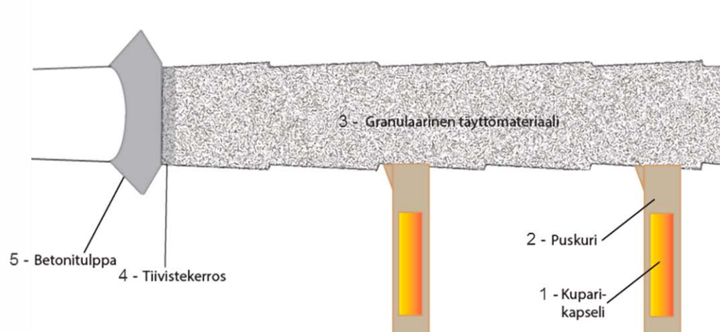
Kuva 17. Tekniset vapautumisesteet: 1 - Loppusijoituskapseli, 2 - Puskuri, 3 - Täyttö (4 - Tiivistyskerros on osa täyttöä), 5 - Loppusijoitustunnelin päätytulppa (ei luokitella tekniseksi vapautumisesteeksi).
