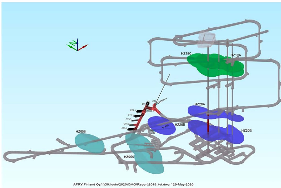
Kuva 3. Paikkamittakaavan merkittävimmät vettäjohtavat hydrogeologiset rakenteet esitettynä ONKALO®:n tunneleita leikkaavina kiekkoina. Rakenteiden värikoodit ovat vihreä: HZ19, tummansininen: HZ20 ja vaaleansininen: HZ056.
