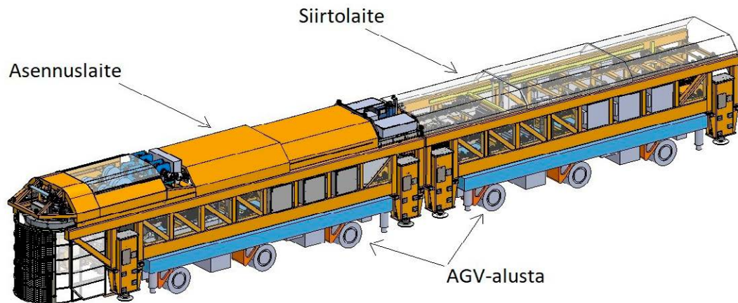
Kuva 10. Puskurilohkojen asennusjärjestelmä
