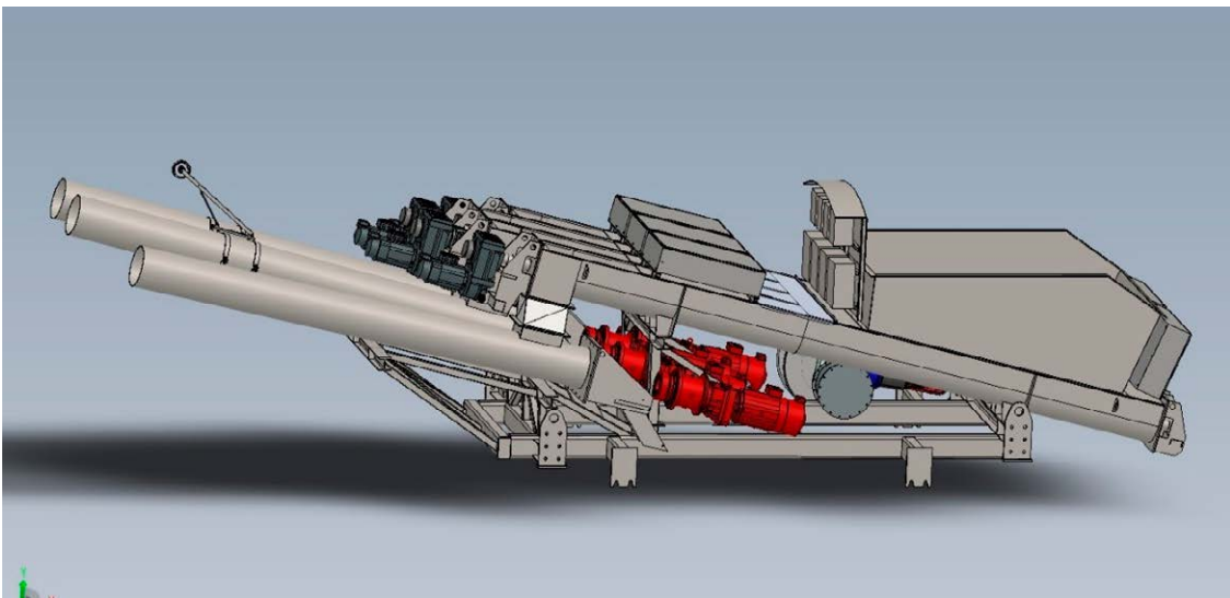
Kuva 11. Tunnelitäytön asennuslaite.
