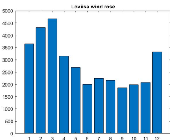
■ Kuva 24. Tuulensuuntajakauma (ns. tuulisuus) Loviisan säämaston mittauksista. Esitetyt Aranon sektorit 1-12 vastaavat 'kellotaulun mukaisia' leviämissuuntia.
