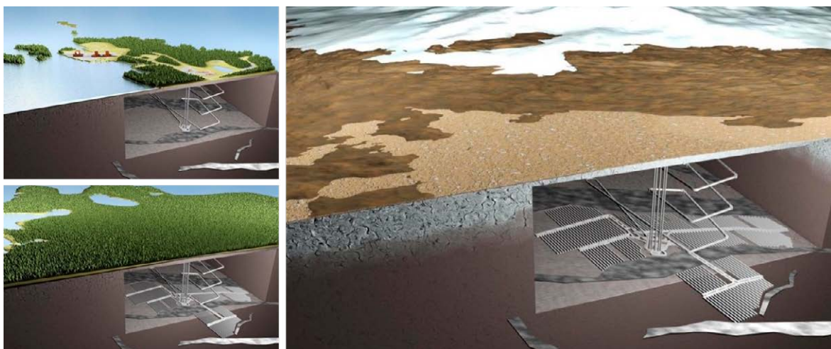
Kuva 22. Olkiluoto ja loppusijoituslaitos (vasemmalla ylhäällä vuonna 2020) tulee olemaan sisämaassa tulevien tuhansien vuosien aikana maankohoamisen vuoksi (vasemmalla alhaalla ~4000 vuoden kuluttua) sekä peittymään mannerjäätikön alle (oikealla ~100 000 vuoden kuluttua).
