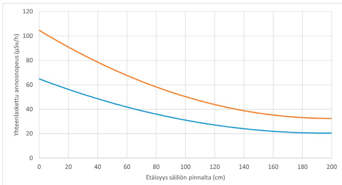
Kuva 15. Yhteenlasketut annosnopeudet (fotonit+neutronit, \mu\text{Sv/h} ) etäisyyden funktiona säiliön pinnasta. Annosnopeus 60 MWd/kgU keskipalamalla on esitetty oranssilla värillä ja 50 MWd/kgU keskipalamalla sinisellä värillä. Molemmissa tapauksissa jäähdytysajaksi on oletettu 20 vuotta.
