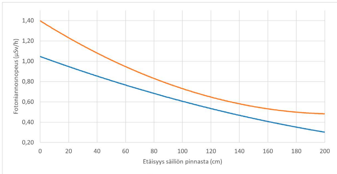
Kuva 12. Lasketut fotoniansnosnopeudet ( \mu\text{Sv/h} ) etäisyyden funktiona säiliön pinnasta. Annosnopeus 60 MWd/kgU keskipalamalla on esitetty oranssilla värillä ja 50 MWd/kgU keskipalamalla sinisellä värillä. Molemmissa tapauksissa jäähtymisajaksi on oletettu 20 vuotta.
