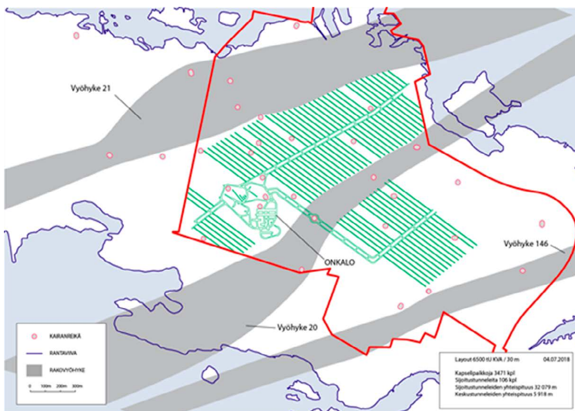
Kuva 3-6. 6500 tU suuruiselle käytetyn polttoaineen määrälle tarkoitetut loppusijoitustilat asemituna asema-alue-alueelle, asema-alueen raja on merkitty punaisella. Kuvassa näkyvät myös tämänhetkisen tiedon mukaiset merkittävimmät sijoittelua rajoittavat kalliorakenteet harmaalla.
