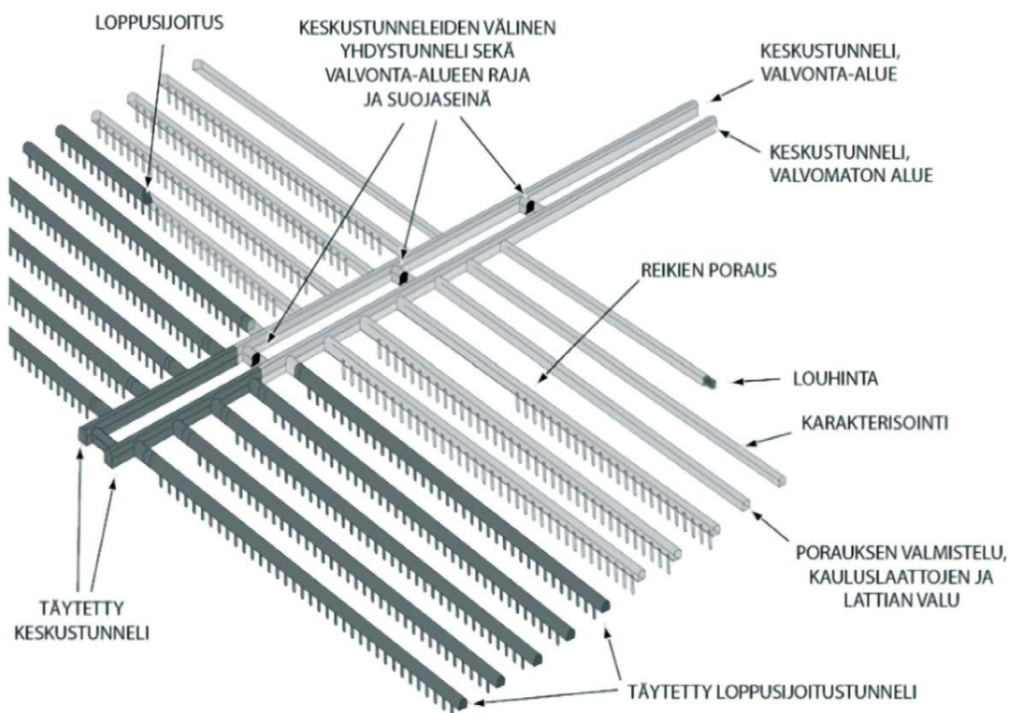
Kuva 3-5. Loppusjoitustunnelien vaiheittainen rakentaminen.
