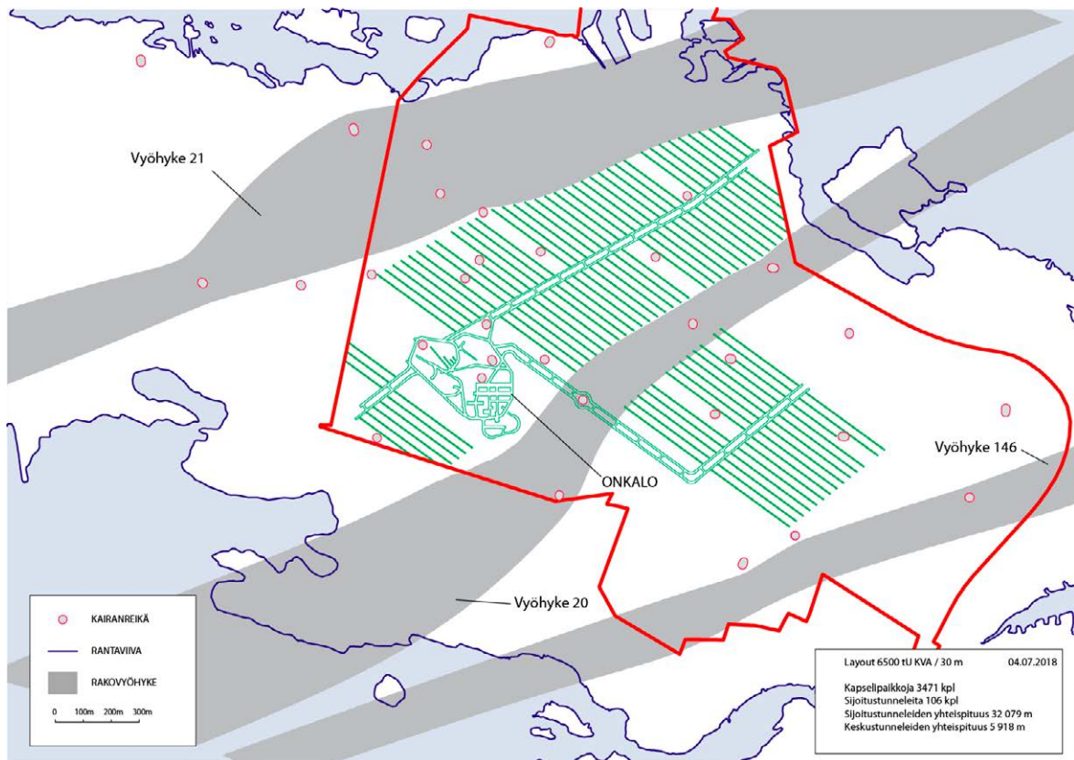
Kuva 3. 6500 tU suuruiseen käytetty polttoaineen määrälle tarkoitettujen loppusijoitustilain asemoina asemakaava-alueella, asemakaava-alueen raja on merkitty punaisella.
