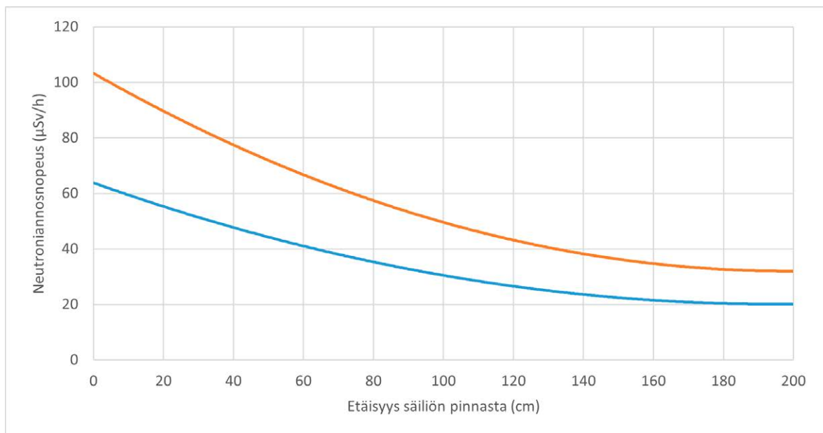
Kuva 13. Lasketut neutroniansnosnopeudet ( \mu\text{Sv/h} ) etäisyyden funktiona säiliön pinnasta. Annosnopeus 60 MWd/kgU keskipalamalla on esitetty oranssilla värillä ja 50 MWd/kgU keskipalamalla sinisellä värillä. Molemmissa tapauksissa jäähtymisajaksi on oletettu 20 vuotta.
