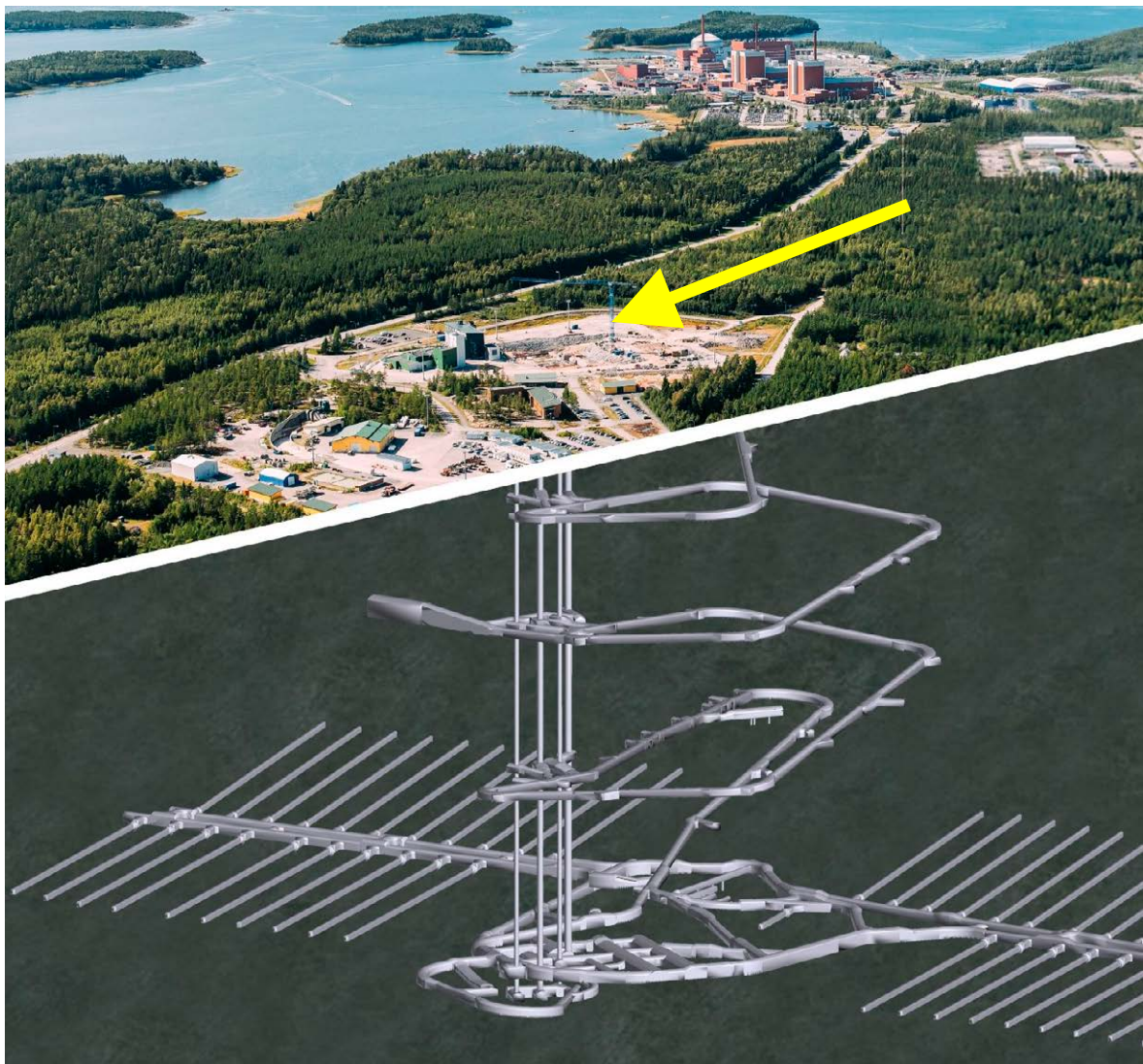
Kuva 1. Kapselointilaitoksella pakataan välivarastolla jäähtynyt käytetty ydinpolttoaine loppusijoituskapseleihin. Kapselointilaitoksesta suljettu kapseli lasketaan kapselihissillä noin 430 metrin syvyyteen loppusijoituslaitokseen, jossa se siirretään loppusijoitusreikään ja peitetään bentoniitilla. Lopuksi tunnelit täytetään ja suljetaan tulpalla. Keltainen nuoli osoittaa kapselointilaitoksen paikkaa (kuvassa rakenteilla).
