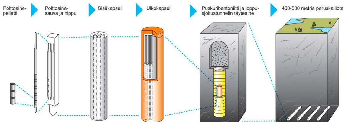
Kuva 15. Loppusijoitusjärjestelmän eri osat moniesteriaatteen mukaisesti.
