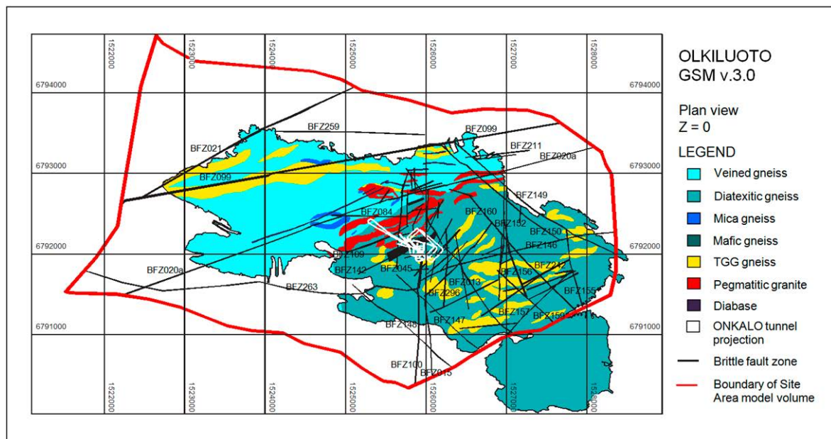
Kuva 6-4. Olkiluodon saaren alueelle tulkitut kallioperän kivilajit ja rikkonaisuusrakenteet.
