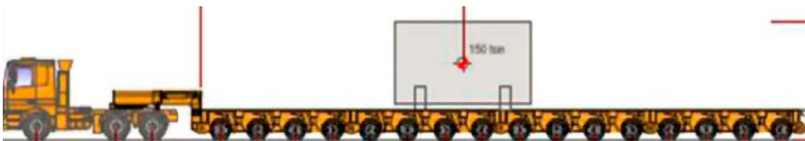
Kuva 4. Loviisan polttoainekuljetukselle soveltuva kuljetuskalustotyyppi (Posiva).
