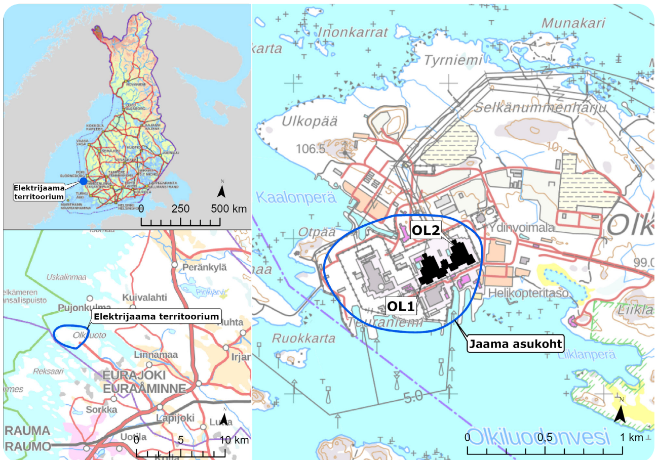
Joonis 2. Olkiluoto elektriijaama territoorium ning tootmisplokkide OL1 ja OL2 asukoht jaama territooriumil.
