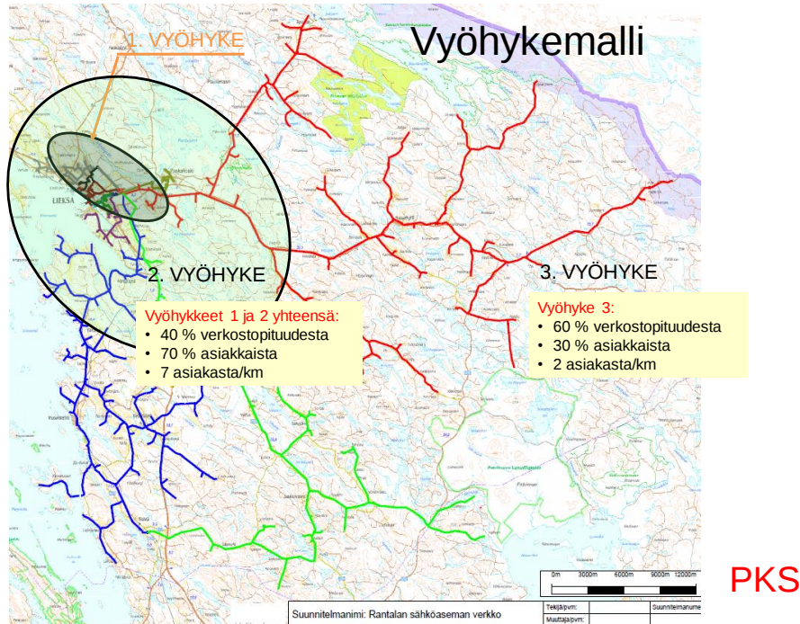
Kuva 5.1 Esimerkki vyöhyketoimintamallista
