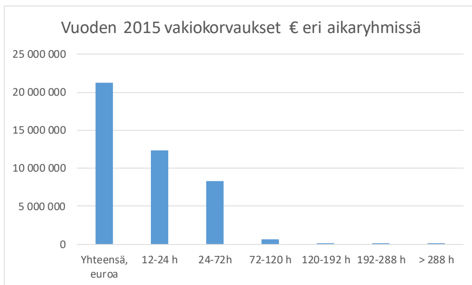
Kuva 6.2 Jakeluverkkoyhtiöiden maksamien vakiokorvausten (€) jakaantuminen keskeytysten pi- tuuden mukaisiin aikaryhmiin vuonna 2015
