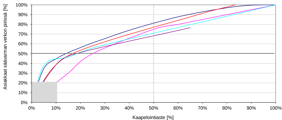
Kuva 4.1 Myrskyvarman verkon piiriin saatavissa olevien sähkönkäyttäjien määrä keskijänniteverkon kaapelointiasteen funktiona muutamissa esimerkkiyhtiöissä. Yhtiöiden alkupisteet on häivytetty.
