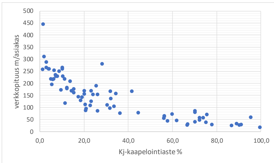
Kuva 4.2 Verkkoyhtiöt kj-kaapelointiasteen ja verkkopituus m/asiakas tunnusluvuilla esitettynä vuonna 2017 /Energiavirasto/
