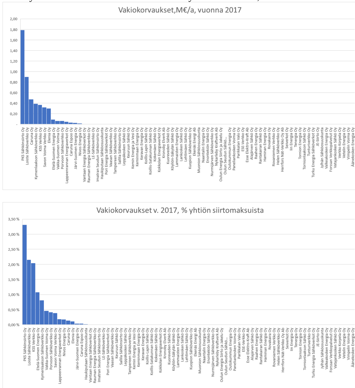
Kuva 6.3 Jakeluverkkoyhtiöiden maksamat vakiokorvaukset yhtiöittäin
