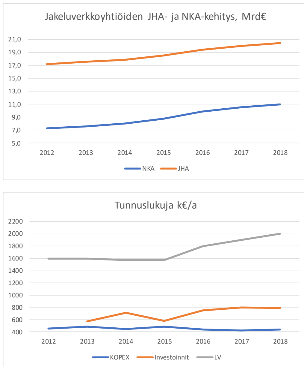
Kuva 2.1 Sähköjakeluverkkoyhtiöiden jälleenhankinta- (JHA) ja nykykäyttöarvojen (NKA), liikevaihdon, investointien ja kontrolloitavien operatiivisten kustannusten kehittyminen vuosina 2012-2018
