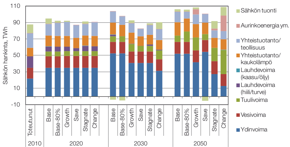
Kuva 4. Sähkönhankinnan rakenne Low Carbon Finland -skenaariossa, TWh.
