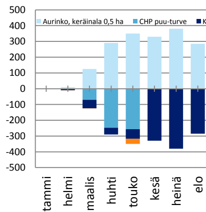
Kuva 29: Aurinkolämmön vaikutus CHP tuotantoon 120 MW puu-turve -kattilalla. [MWh]
