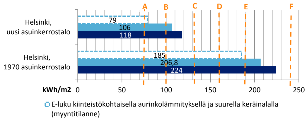
Kuva 9 E-luvut sekä uuden energiatodistusasetuksen mukaiset energialuokat työssä tyyppitaloina käytetyille asuinkerrostaloille ilman aurinkolämpöä sekä aurinkolämmön kanssa. Keskitettyä aurinkolämmön tuotantoa ei huomioida E-luvun laskennassa.
