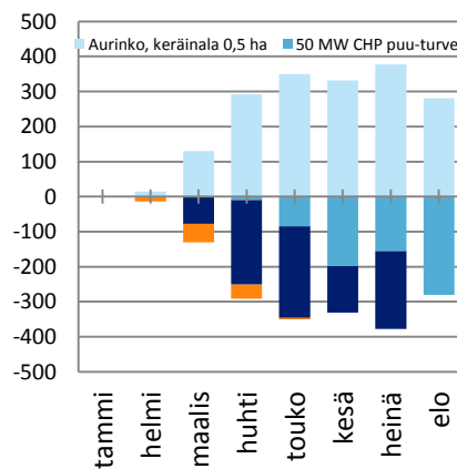
Kuva 30: Aurinkolämmön vaikutus CHP tuotantoon 50 MW puu-turve -kattilalla. [MWh]
