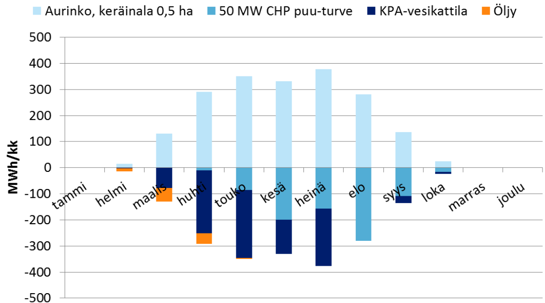
Kuva 15 Aurinkolämmön vaikutus tuotantoon esimerkkitapauksessa 50 MW puu-turve CHP, kun aurinkolämpöä tuotetaan 0,5 ha keräinalalla
