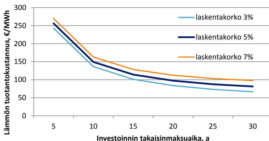
Kuva 6 Aurinkolämmön tuotantokustannuksen herkkyys investoinnin takaisinmaksuajan ja laskentakoron suhteen (Jyväskylä, suuri keräinala, uusi asuinkerrostalo)
