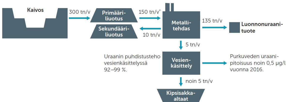
Kuva 3. Kaivoksen uraanitase kun uraanin talteenottolaitos on käytössä.
