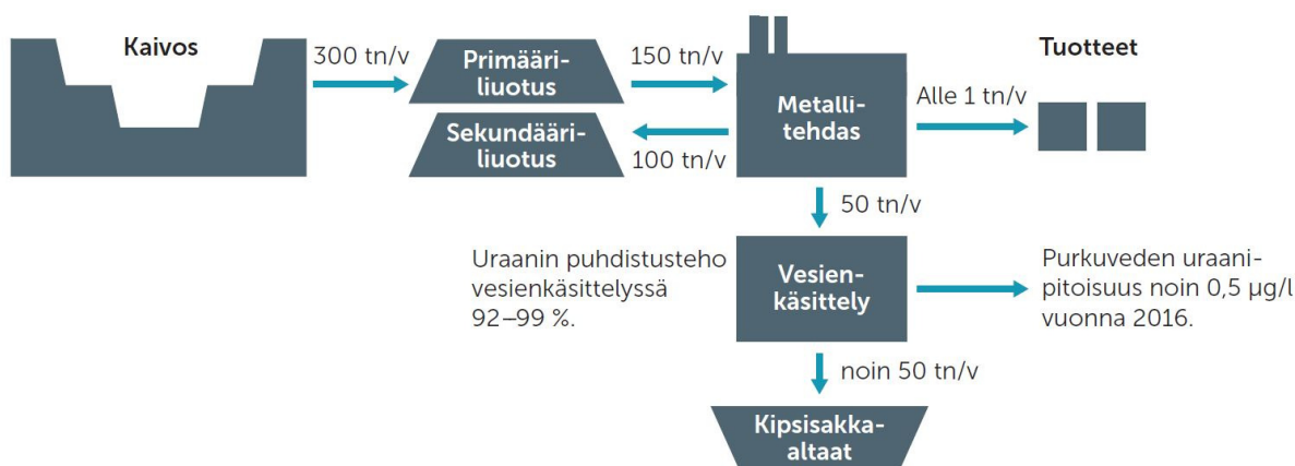
Kuva 2. Kaivoksen uraanitase ilman uraanin talteenottoa.
